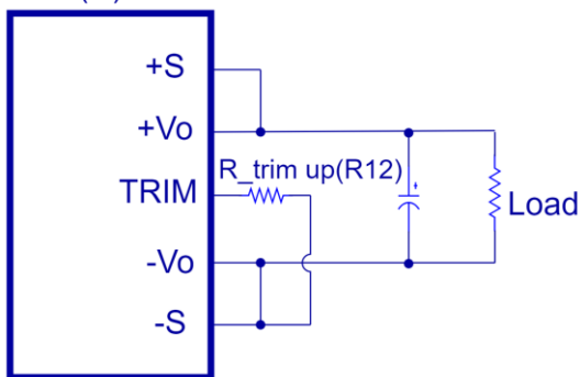
CMFC(D) Module
